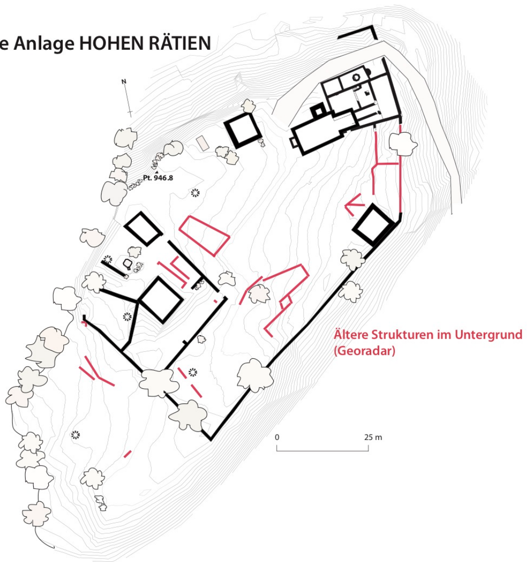
Abbildung 3: Aufnahme mit Georadar
